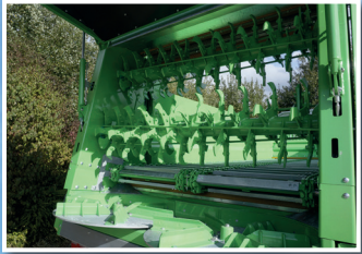
2 horizontale Fräswalzen mit Streuteller (2 x ø 1040 mm)
