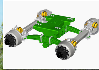
Bogie Roll-Over con eje seguidor
