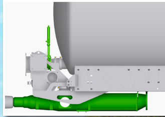
Bomba helicoidal con recoge-piedras y pre-equipamiento Jumbo frontal
